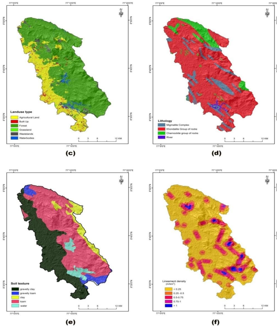
Fig. 2. (c) Land use (d) Lithology (e) Soil texture (f) Lineament density
